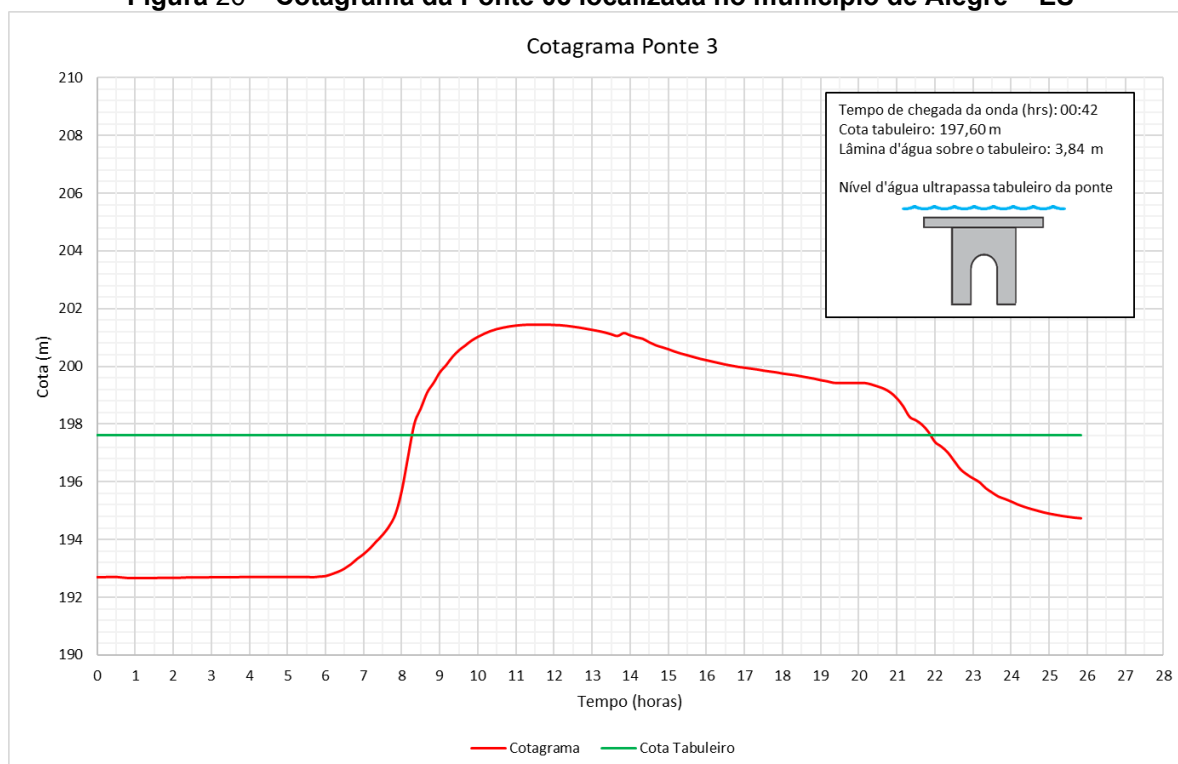
Figura 26 – Cotagrama da Ponte 03 localizada no município de Alegre – ES
