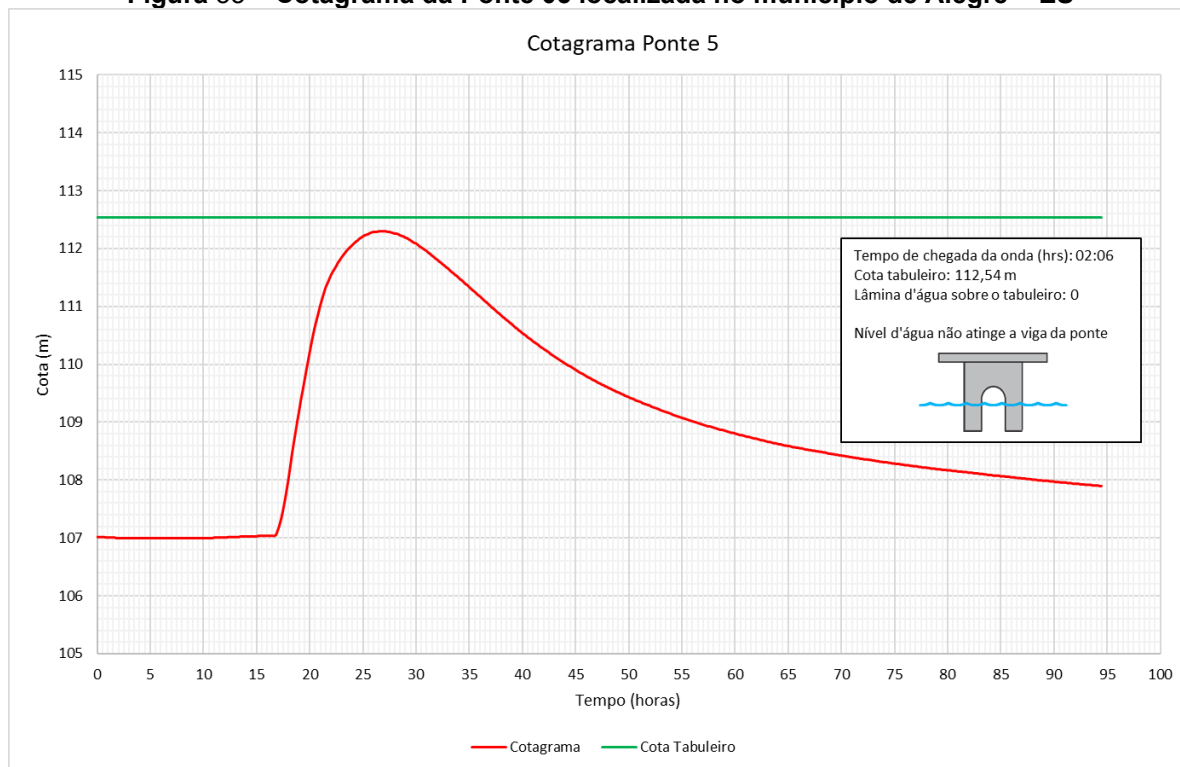
Figura 35 – Cotagrama da Ponte 05 localizada no município de Alegre – ES
