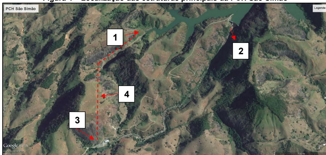
Figura 4 – Localização das estruturas principais da PCH São Simão
