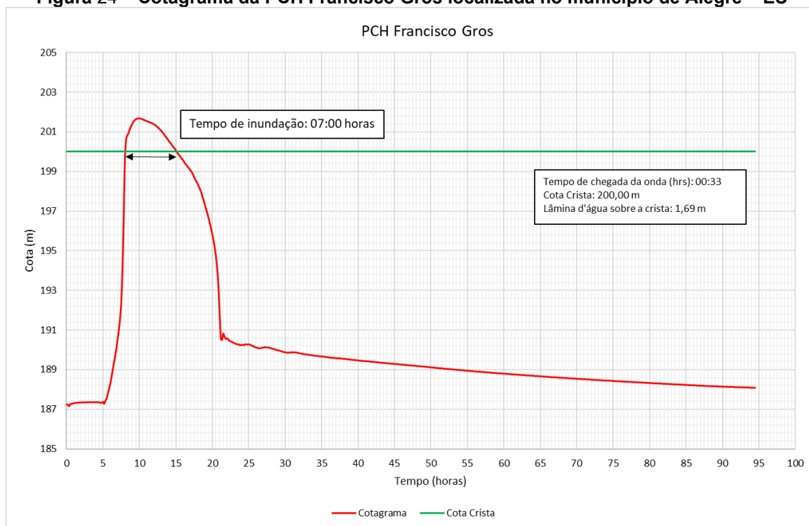
Figura 24 – Cotagrama da PCH Francisco Gros localizada no município de Alegre – ES
