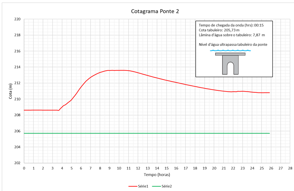
Figura 22 – Cotagrama da Ponte 02 localizada no município de Alegre – ES
