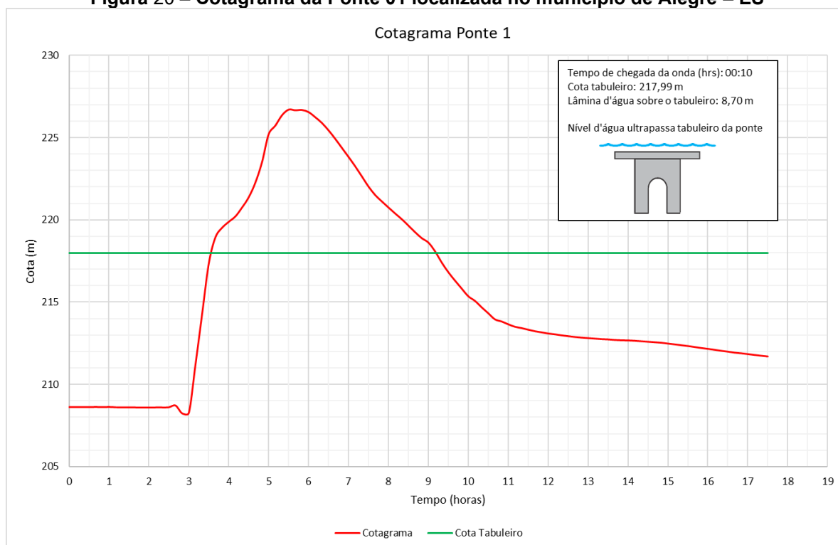
Figura 20 – Cotagrama da Ponte 01 localizada no município de Alegre – ES
