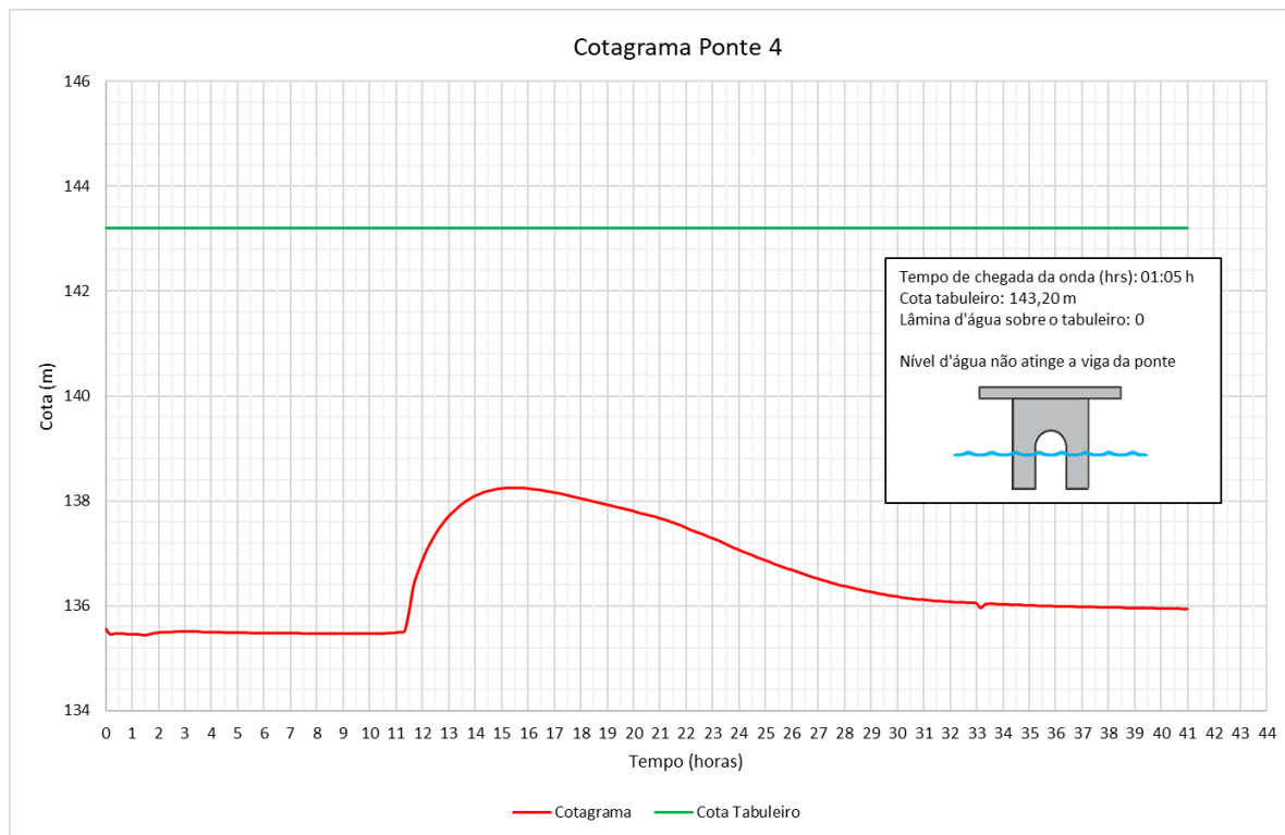
Figura 33 – Cotagrama da Ponte 04 localizada no município de Alegre – ES
