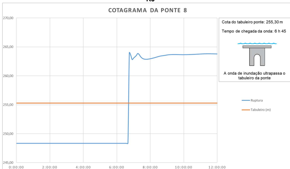
Figura 61– Cotagrama da Ponte 08 localizada entre os municípios de Chiador - MG e Três Rios – RJ
