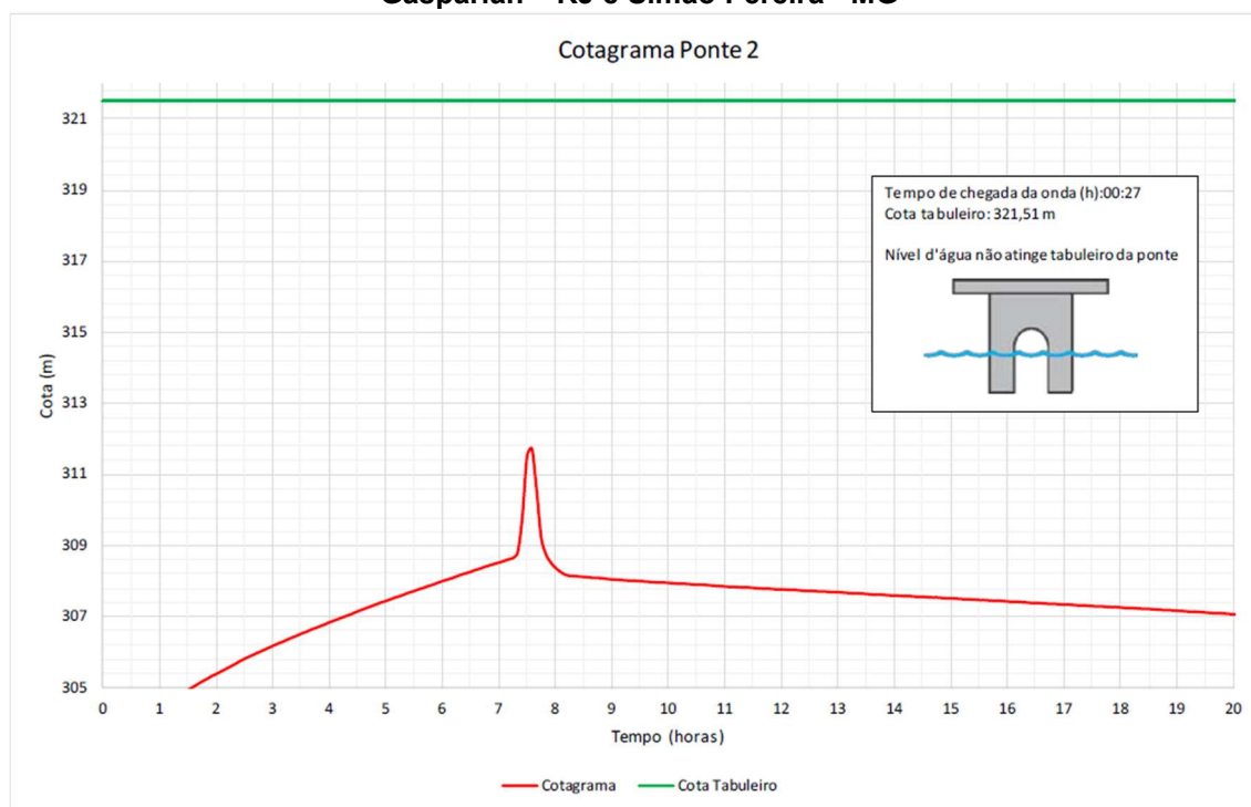
Figura 19 – Cotagrama da Ponte 02 (Rodovia BR040) localizada entre os municípios de C. Levy Gasparian – RJ e Simão Pereira - MG
