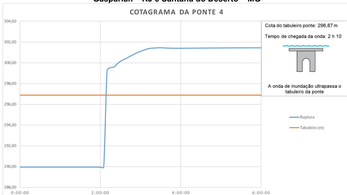
Figura 49– Cotagrama da Ponte 04 localizada entre os municípios de Comendador Levy Gasparian – RJ e Santana do Deserto – MG
