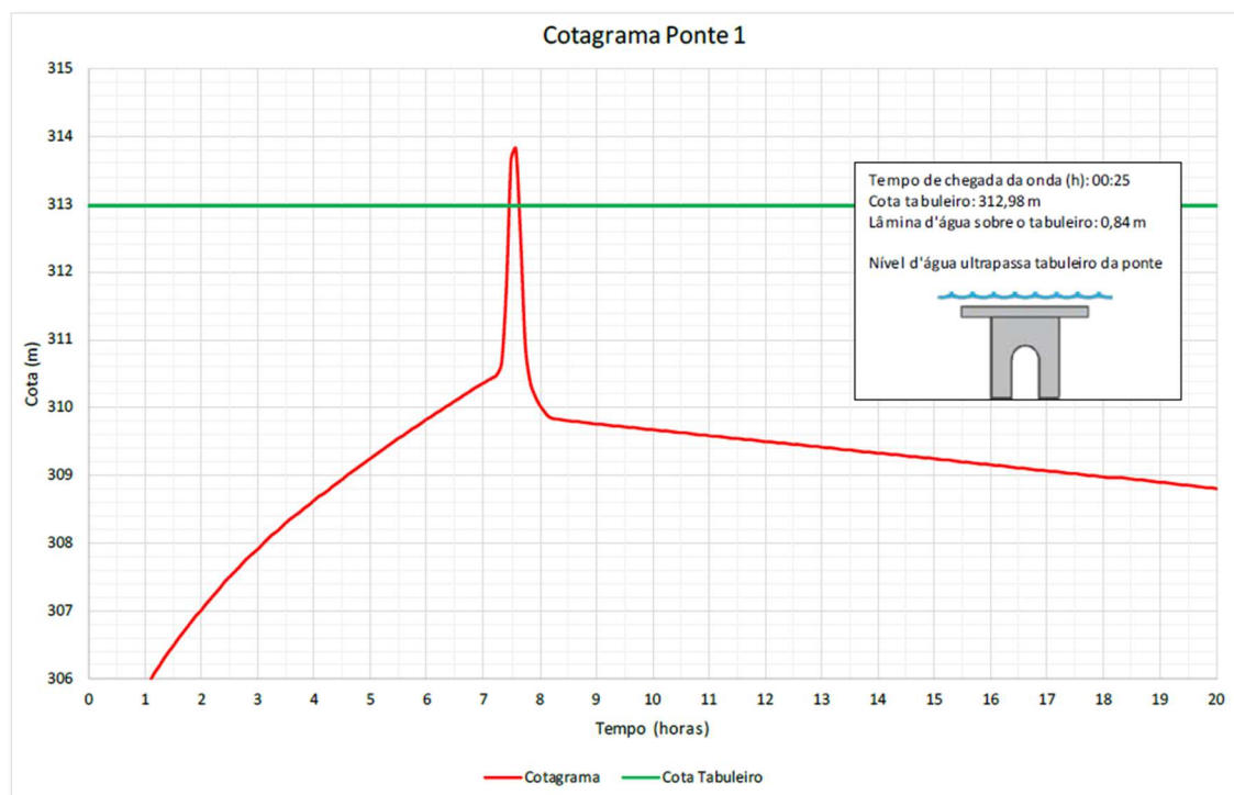
Figura 17 – Cotagrama da Ponte 01 localizada entre os municípios de C. Levy Gasparian – RJ e Simão Pereira - MG
