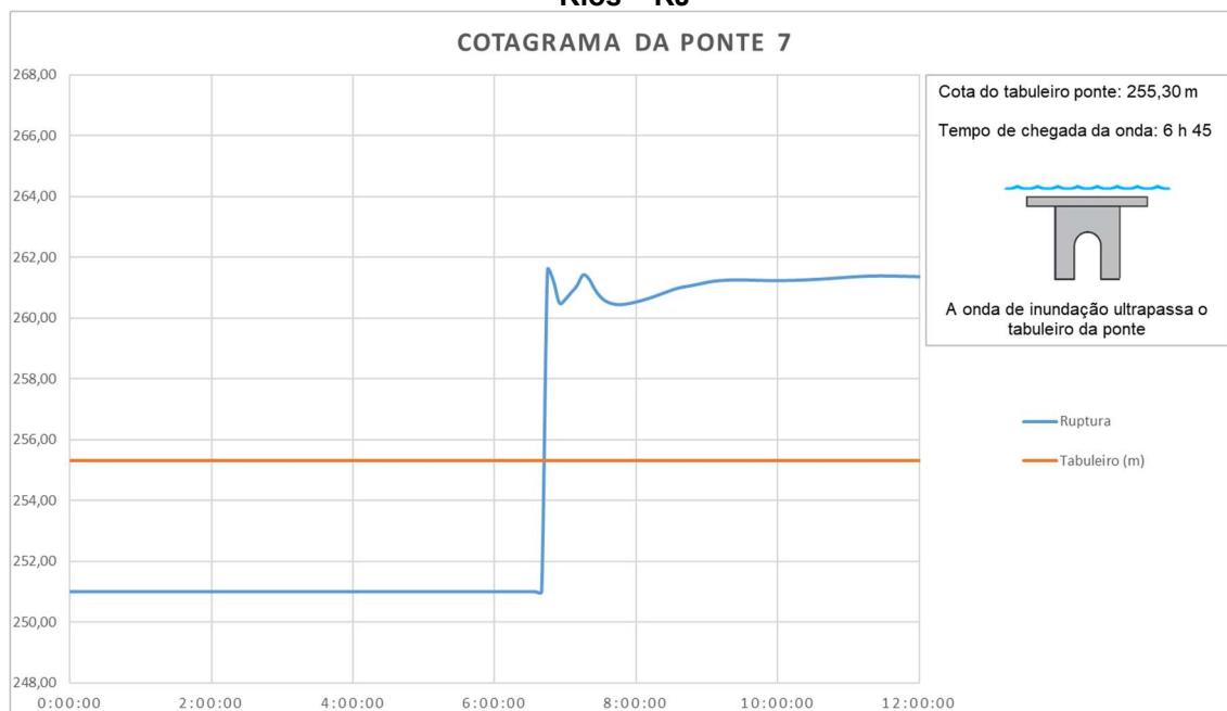
Figura 60 – Cotagrama da Ponte 07 localizada entre os municípios de Chiador - MG e Três Rios – RJ
