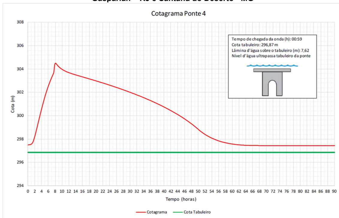
Figura 23 – Cotagrama da Ponte 04 localizada entre os municípios de Comendador Levy Gasparian – RJ e Santana do Deserto - MG
