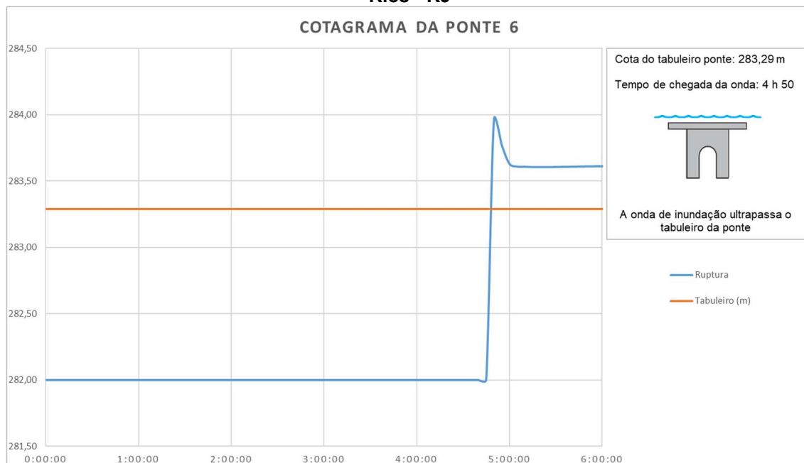
Figura 59– Cotagrama da Ponte 06 localizada entre os municípios de Chiador – MG e Três Rios - RJ
