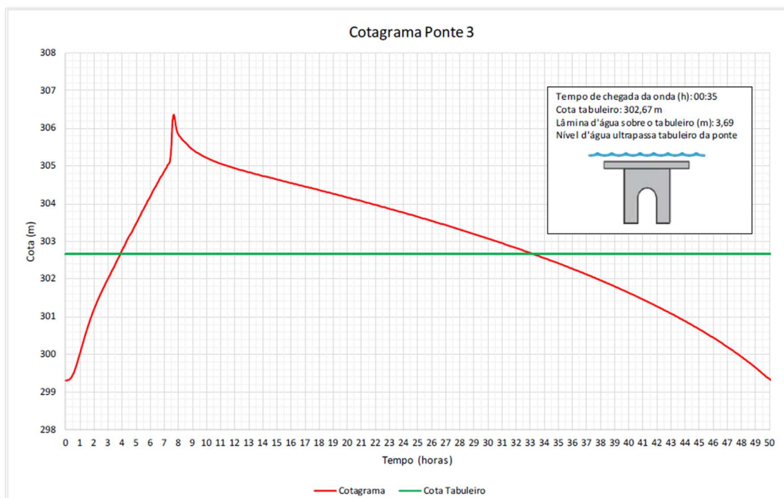
Figura 21 – Cotagrama da Ponte 03 localizada entre os municípios de C. Levy Gasparian – RJ e Simão Pereira – MG
