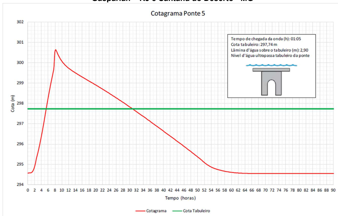
Figura 25 – Cotagrama da Ponte 05 localizada entre os municípios de Comendador Levy Gasparian – RJ e Santana do Deserto - MG
