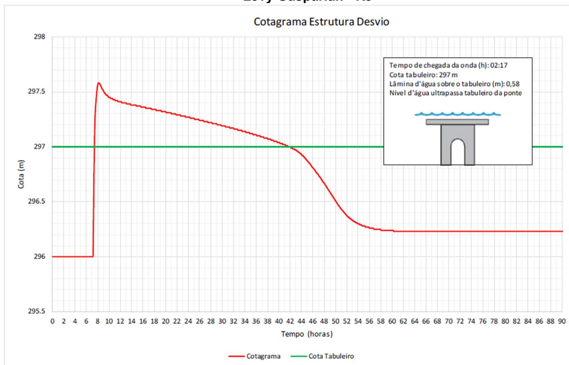
Figura 35 – Cotagrama da Estrutura do Desvio da PCH Santa Fé, município de Comenador Levy Gasparian - RJ
