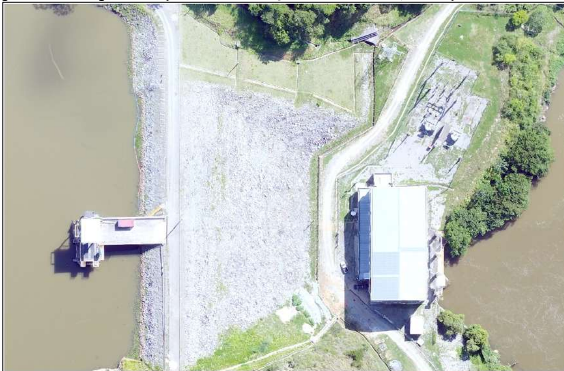
Figura 39 – Barragem Principal e Casa de Força da PCH Santa Fé, município de Três Rios - RJ
