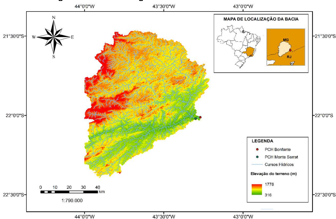
Figura 3 – Bacia Hidrográfica Contribuinte da PCH Bonfante
