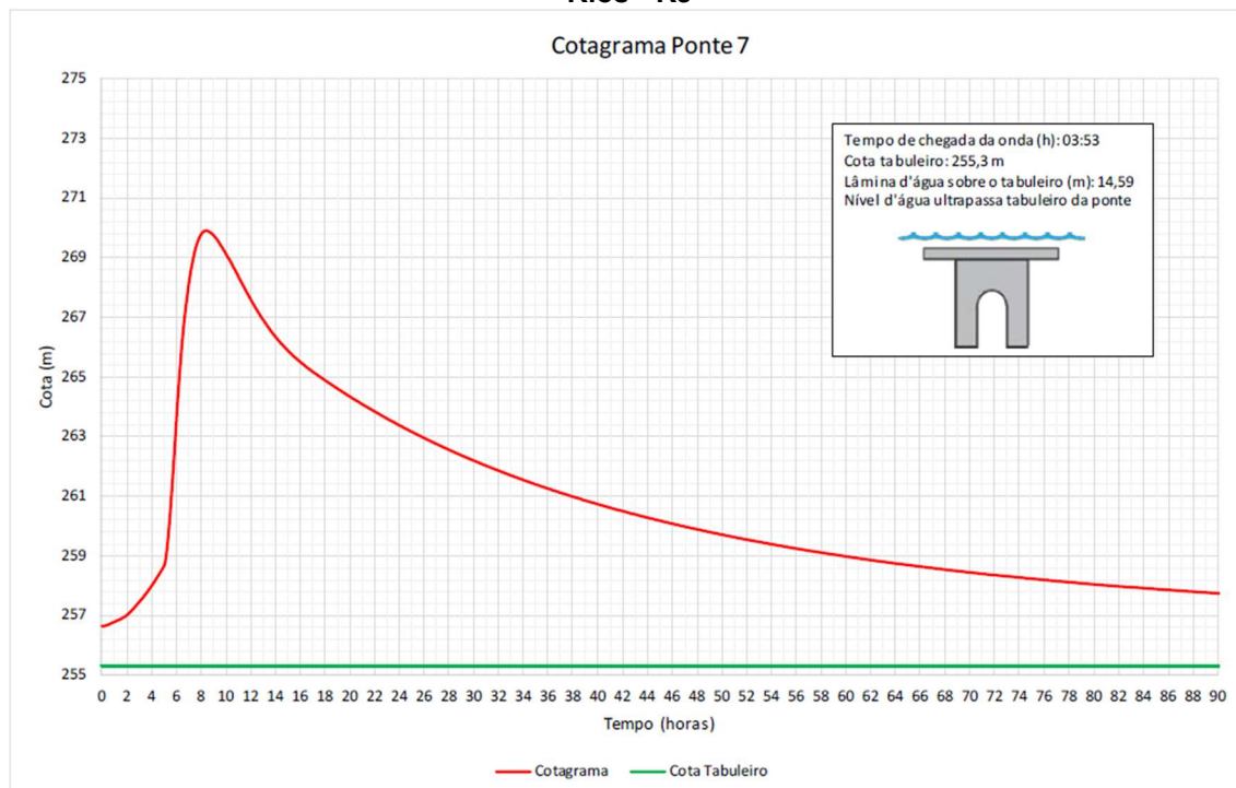
Figura 40 – Cotagrama da Ponte 07 localizada entre os municípios de Chiador – MG e Três Rios - RJ
