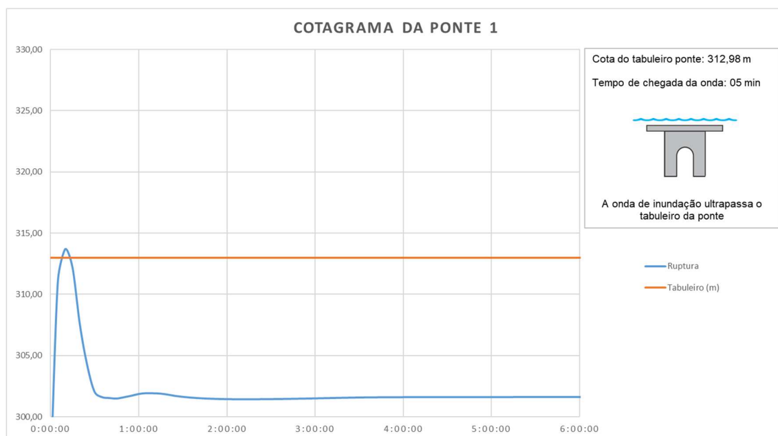
Figura 47 – Cotagrama da Ponte 02 (Rodovia BR040) localizada entre os municípios de C. Levy Gasparian - RJ e Simão Pereira – MG
