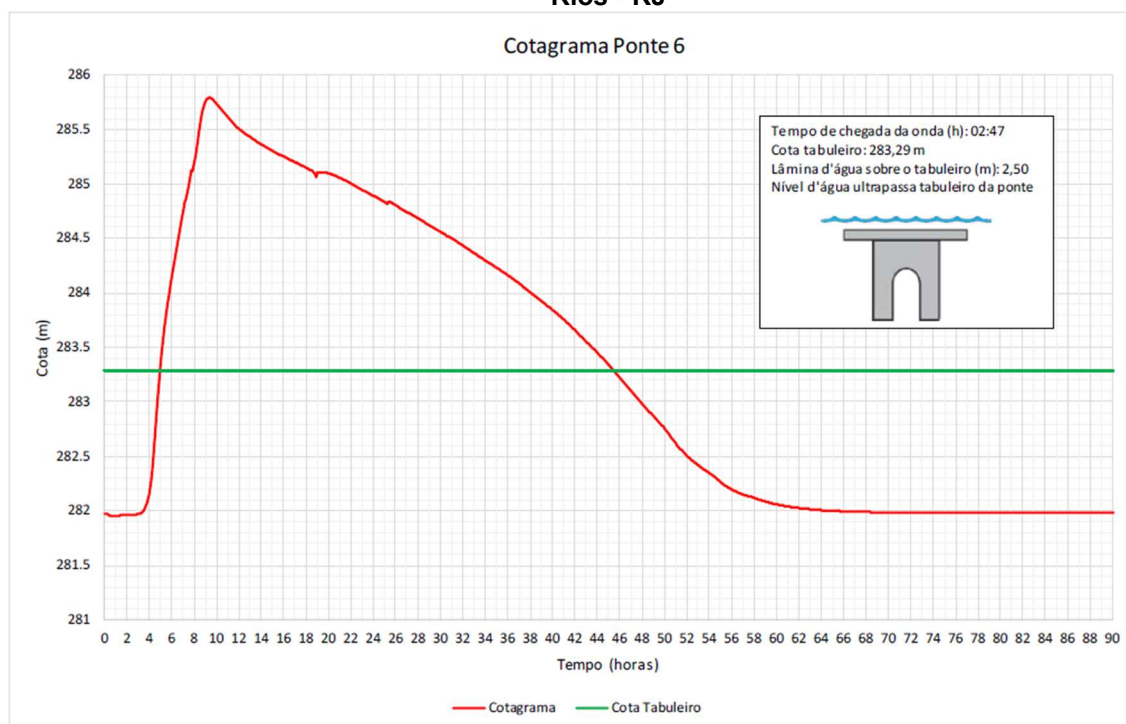
Figura 37 – Cotagrama da Ponte 06 localizada entre os municípios de Chiador – MG e Três Rios - RJ
