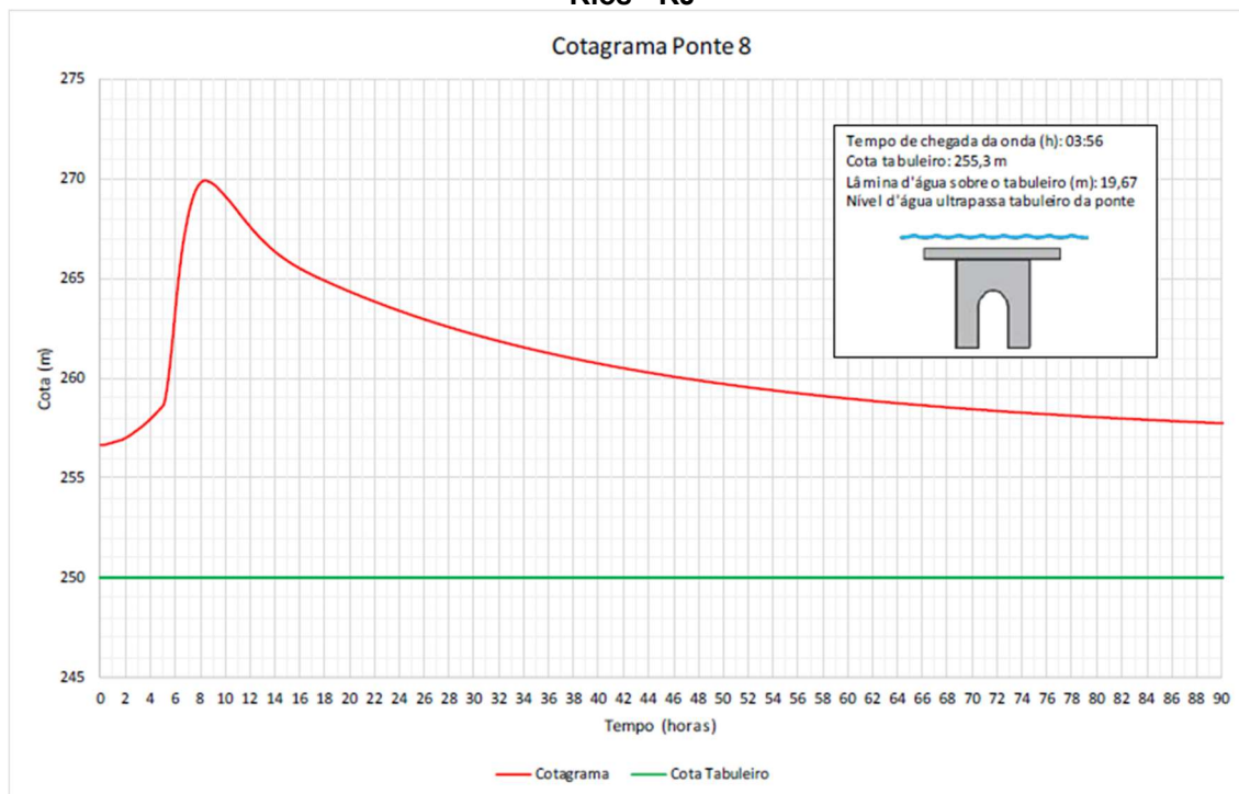
Figura 42 – Cotagrama da Ponte 08 localizada entre os municípios de Chiador – MG e Três Rios - RJ
