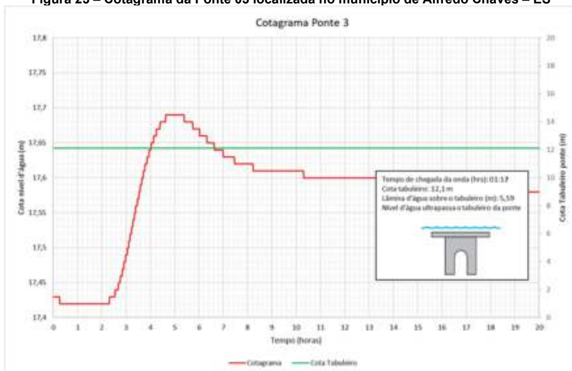
Figura 23 – Cotograma da Ponte 03 localizada no município de Alfredo Chaves – ES
