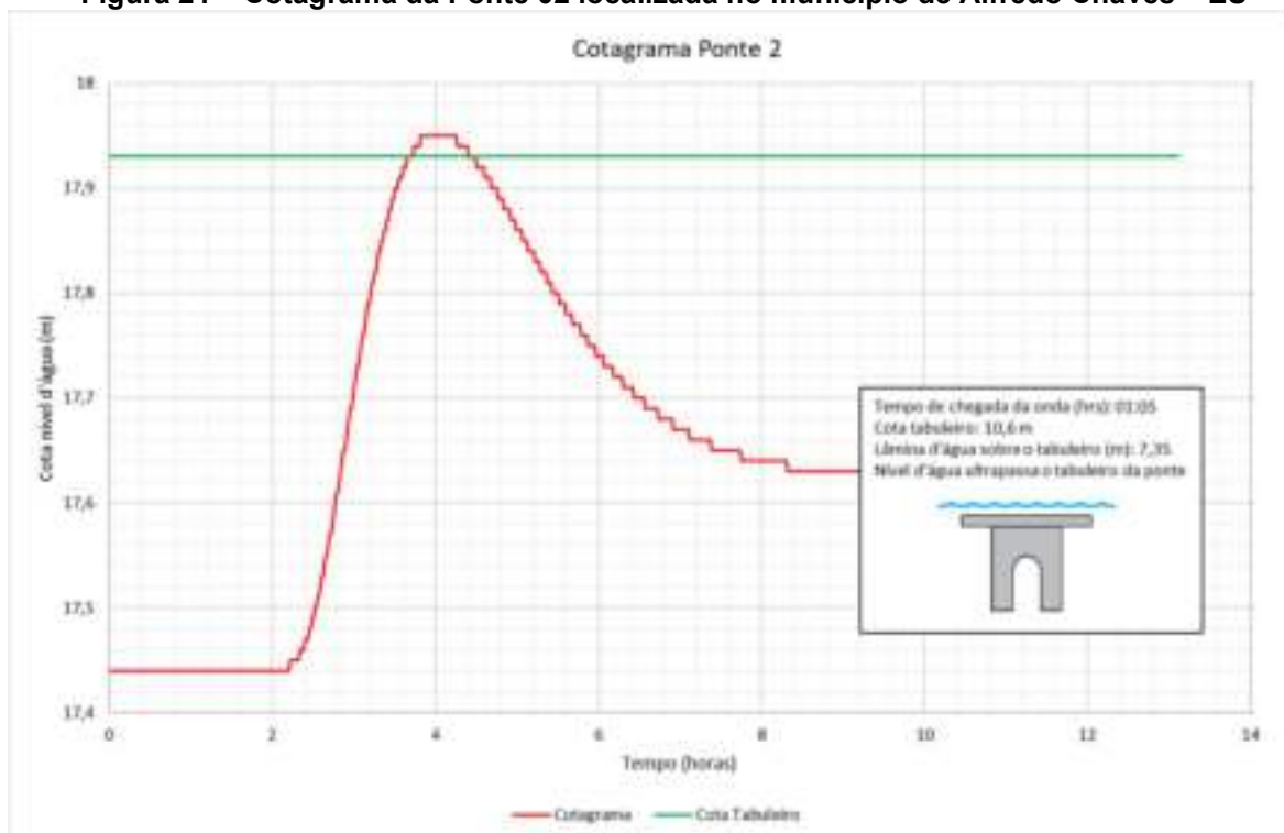
Figura 21 – Cotograma da Ponte 02 localizada no município de Alfredo Chaves – ES
