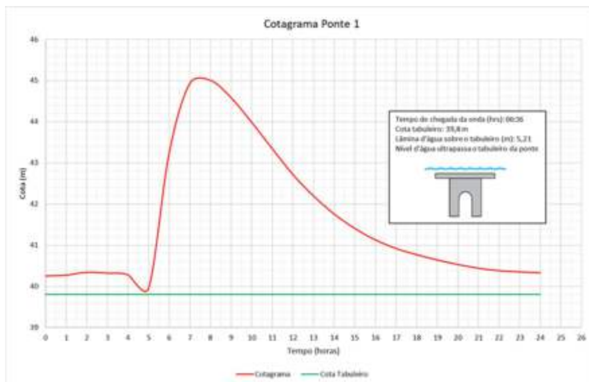
Figura 19 – Cotograma da Ponte 01 localizada no município de Alfredo Chaves – ES
