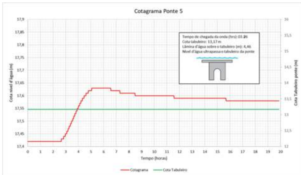
Figura 27 – Cotograma da Ponte 05 localizada no município de Alfredo Chaves – ES
