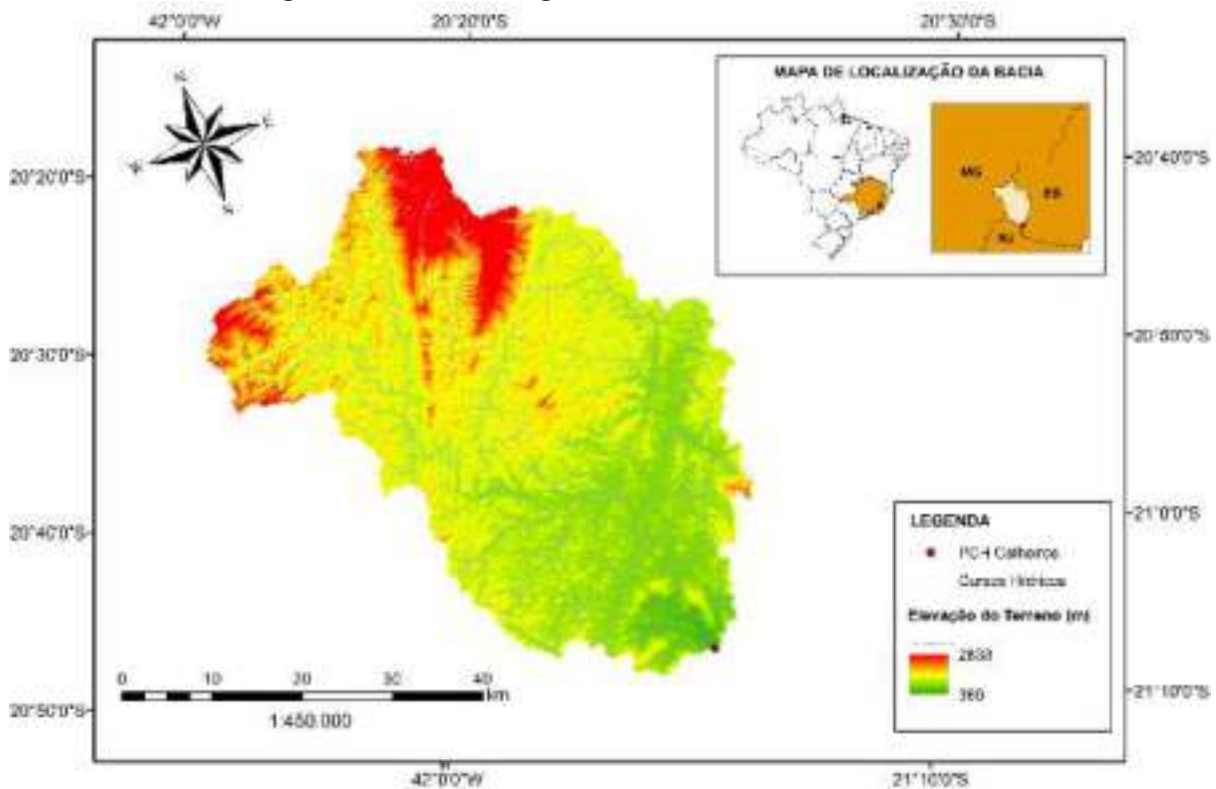
Figura 3 – Bacia Hidrográfica Contribuinte da PCH Calheiros
